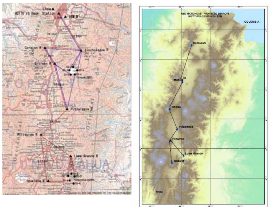
Red de microondas
